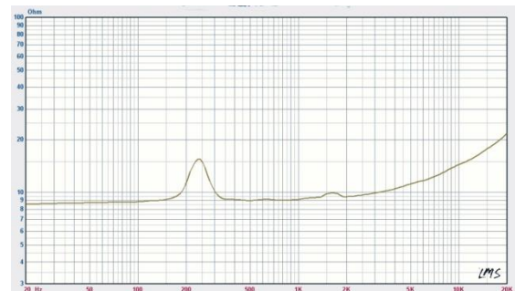
Impedanz-Frequenzgang
